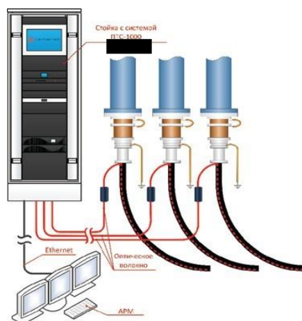
Рисунок 19. Пример интеллектуальной системы контроля температуры высоковольтных кабельных линий на основе распределенного
